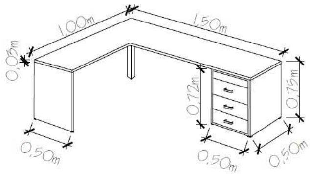
VISTA - MESA EM L
