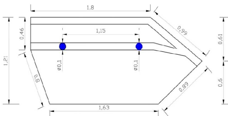
VISTA LATERAL - CAIXA DE ENTULHO COM CAPACIDADE DE 4M 3 . LARGURA DA CAIXA DE ENTULHO: 1,60 M.
